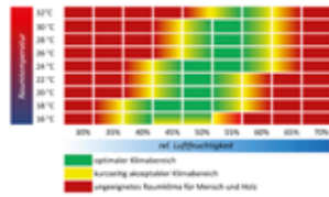
Behaglichkeitsdiagramm
