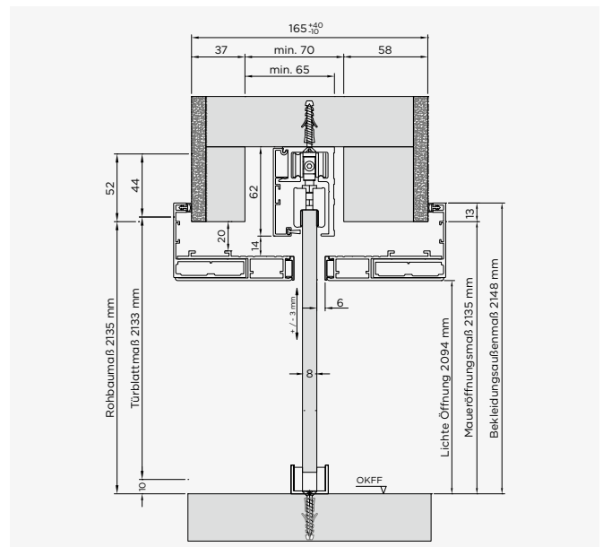
Höhenschnitt Türblatt: 8–9 mm Ganzglastür Beschlag: vorgel. für licht & harmonie Schiebetürsystem Tvin 2.0 | 120 In-Wand laufend
