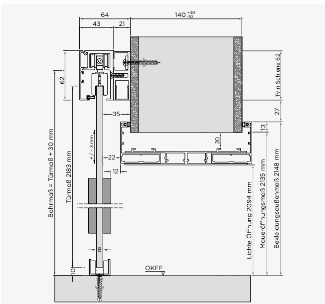
Höhenschnitt Türblatt: 8–9 mm Ganzglastür Beschlag: licht & harmonie Schiebetürsystem Tvin 2.0 vor Zarge
