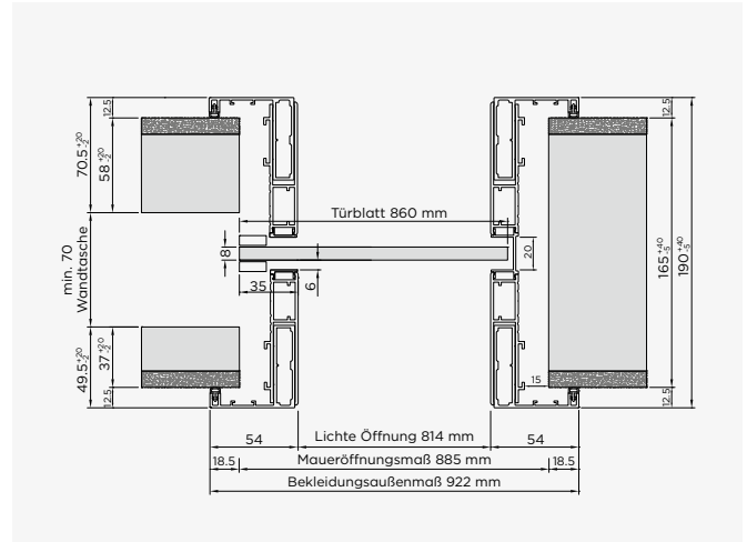
Türblatt: 8–9 mm Ganzglastür Beschlag: vorgel. für licht & harmonie Schiebetürsystem Tvin 2.0 | 120 In-Wand laufend
