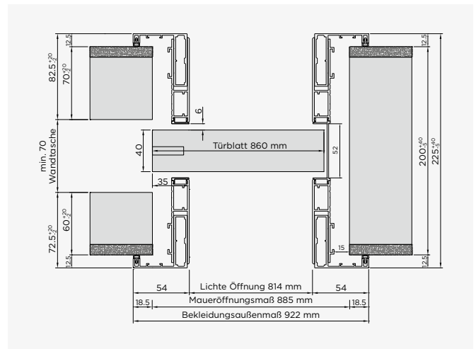
Türblatt: 40 mm Holztür Beschlag: vorgel. für licht & harmonie Schiebetürsystem Tvin 2.0 | 120 In-Wand laufend
