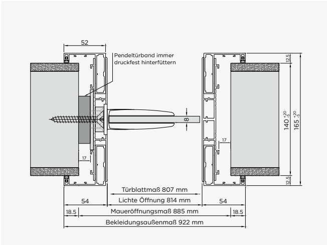
Türblatt: 8–9 mm Ganzglastür Beschlag: licht & harmonie Pendeltürband Swing 2.0
