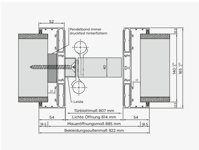
Türblatt: 40 mm Holztür Beschlag: Pendeltürband Fridavo 39
