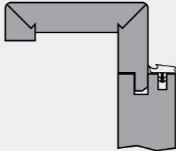
4 ZARGE MIT KLEINER RUNDKANTE FRAME WITH SMALL ROUNDED EDGE
