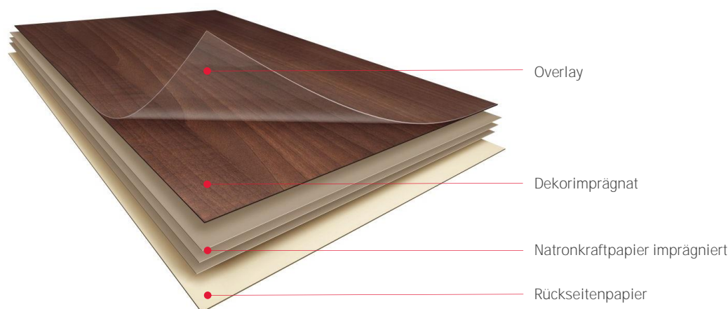
Schichtstoffaufbau MED – Nennstärke 0,80 mm
